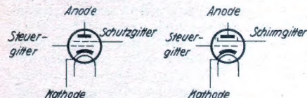
Abb. 1. Das Röhren-Schaltzeichen, das jedem Amateur geläufig sein muß und was es enthält.
