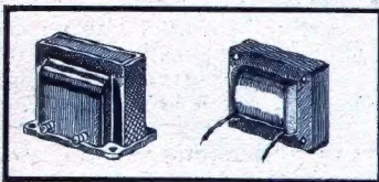
Der Transformator in der Praxis befindet sich meist in einem Gehäuse aus Isoliermaterial oder in einer Blechverfälschung, wie links dargestellt. Er besitzt 4 Klemmen, 2 für die Primärwicklung und 2 für die Sekundärwicklung. Rechts der Eisenkern mit der Spule.
