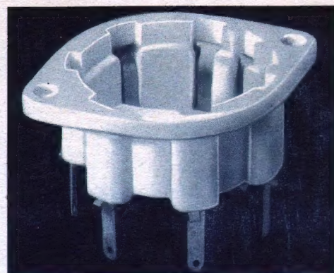
Eine der neuen Fassungen aus keramischem Isoliermaterial. Wir erkennen die Kontaktfedern, die an die stiftlosen Röhrenkontakte drücken.
