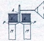
Abb. 1. Beim Freischwinger schwingt der Anker frei vor den Polen. Ein Anker schlägt an die Pole ist deshalb ausgeföhren.
