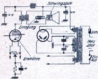
Abb. 6. Die Erregerleistung für den Lautsprecher entnimmt man zweckmäßig dem Gleichrichterteil des Empfängers, vorausgesetzt, daß er hoch genug belastbar ist. Die Schaltung zeigt, wie Netzteil und Erregungspule in diesem Fall zu schalten sind.
